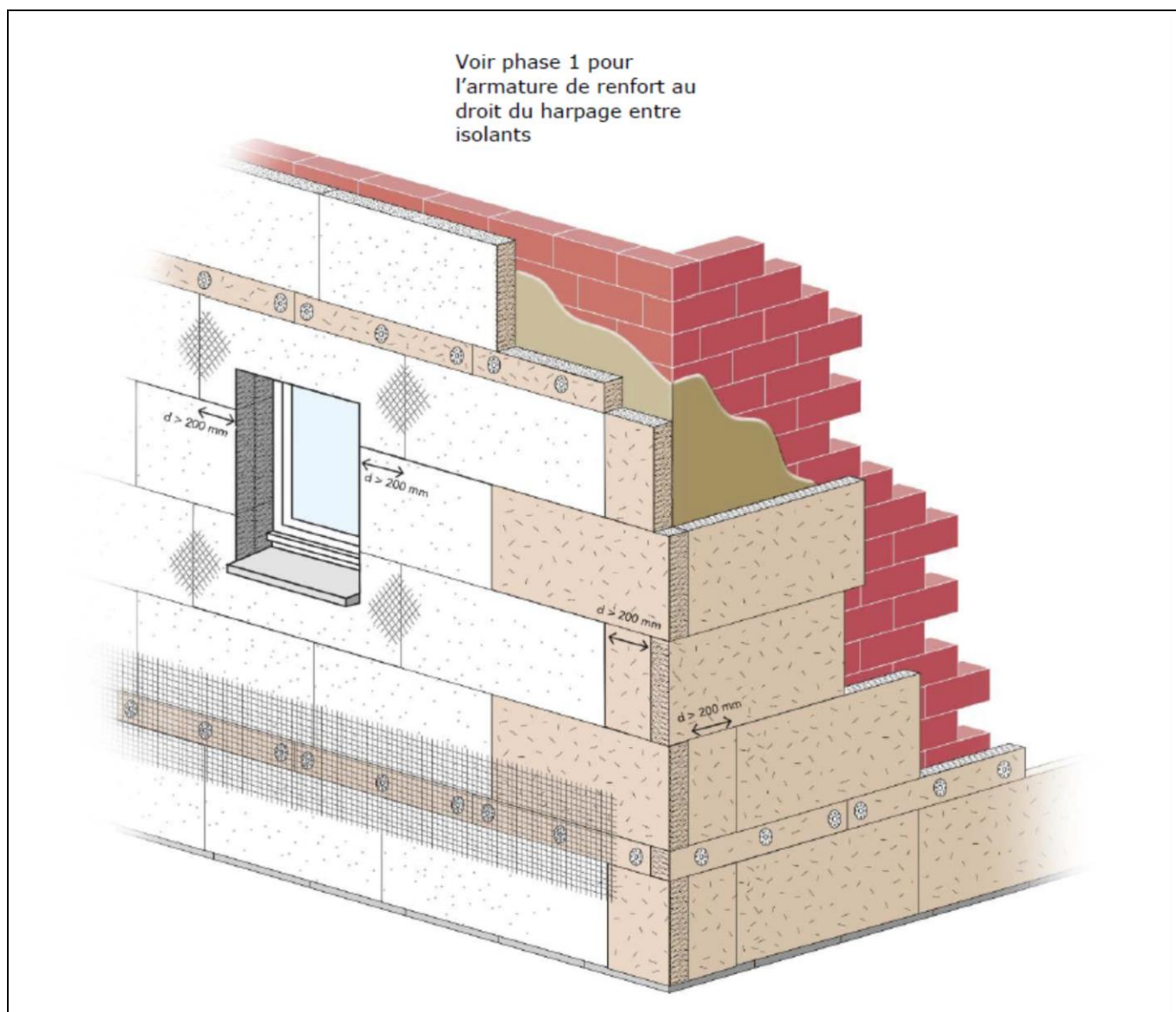
Phase 3 : Pose de l'armature en partie courante
